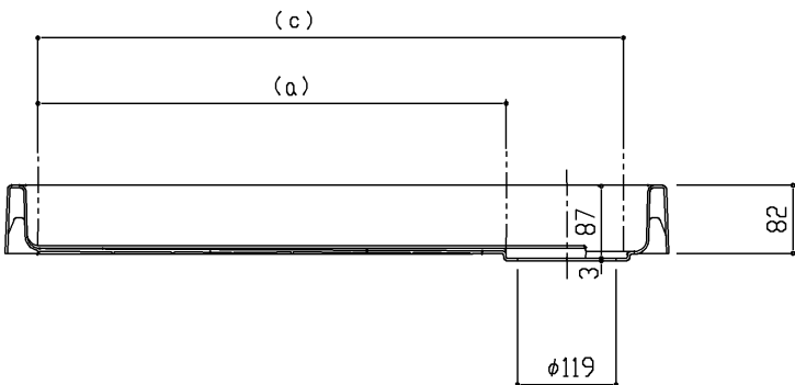
断面A-A
